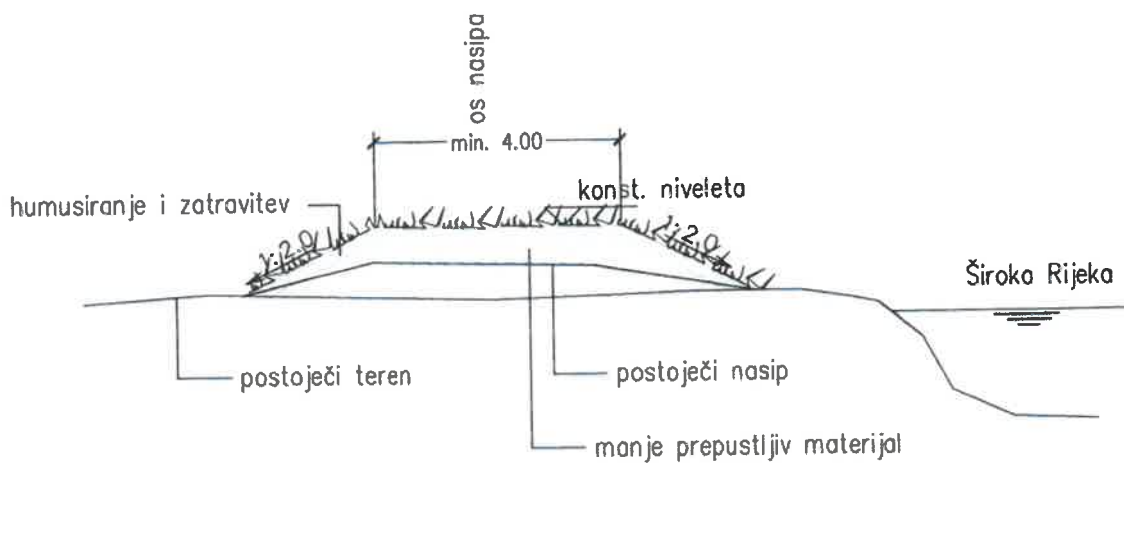
Slika 2: presjek nasipa
